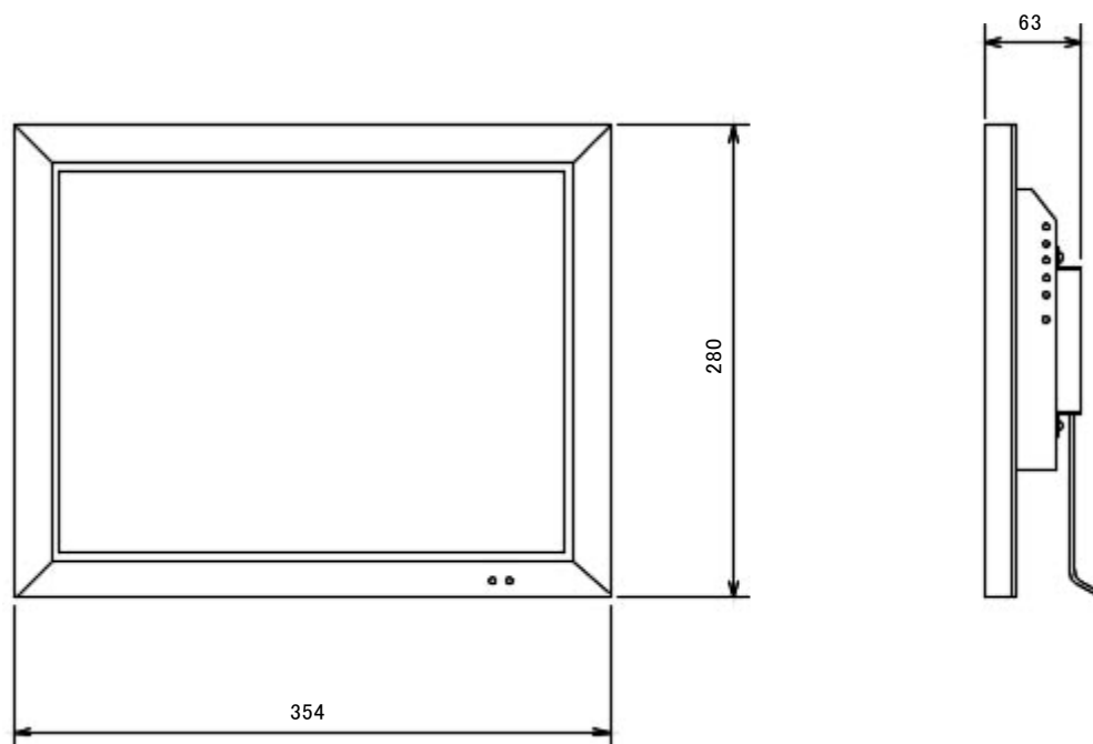
外形寸法図/NM-LCD155A
